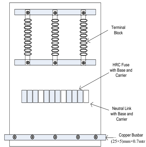
132 & 33KV CVT/PT Console Box i) TB: 30 Nos.(10×3) ii) 16A 415V AC Fuse: 09 Nos. iii) 16A 415V AC Neutral Link Base with Carrier: 03 Nos.
